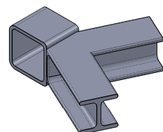
Z-11 Widok: B Ilość: 4
