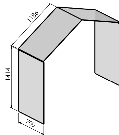
PW-1 Dach, Ściana Widok ogólny Ilość: 3
