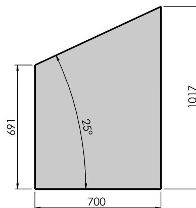
PL-3 Front góra Widok ogólny Ilość: 4
